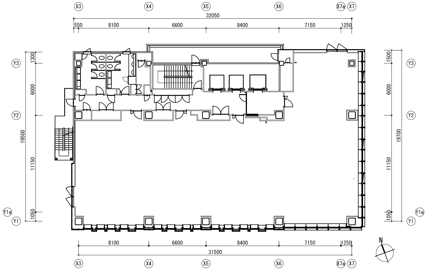
基準階6~10階 平面図 S=1/250
